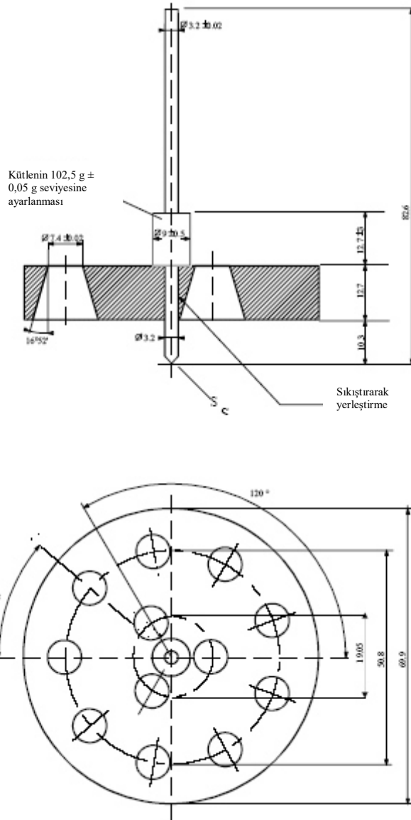
Şekil 1 - Penetrometre
